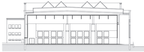
Querschnitt 1:850
